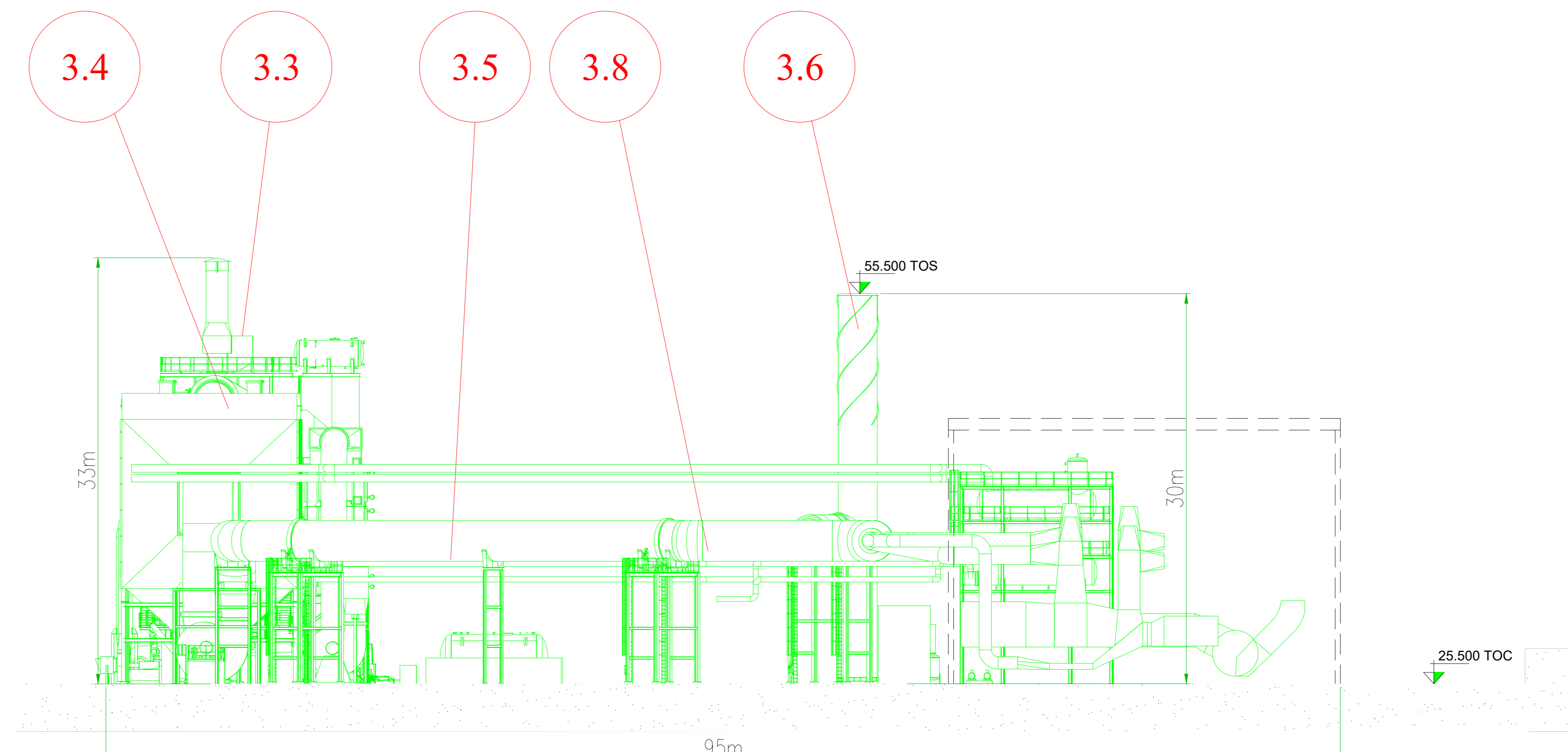
Section D-D
